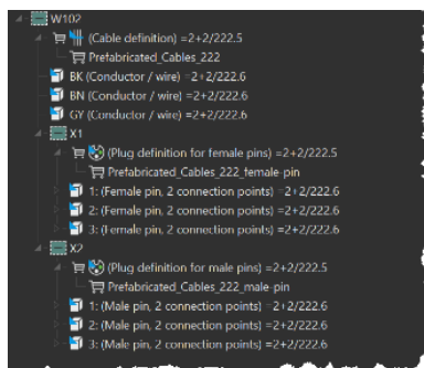
Abbildung 6: Platziertes vorkonfektionierte Kabel mit Artikeln im Betriebsmittel-Navigator.
